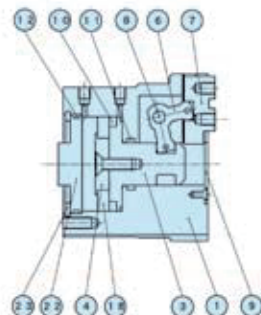
CKA-20AS 标准型
