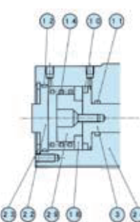
CKA-20AS 常开型
