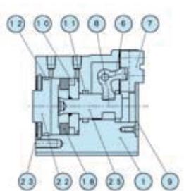
CKA-25AS~40AS 标准型
