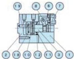
CKA-20AS 标准型
