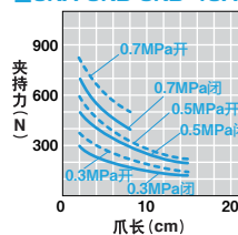
■CKA·CKB·CKD-40AS
