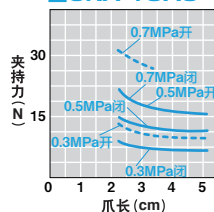
■CKA-15AS
