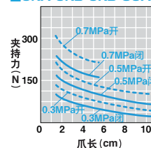
■CKA·CKB·CKD-30AS
