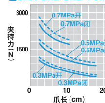
■CKA·CKB·CKD-70MS
