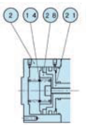
CKA-50MS~70MS 常开型
