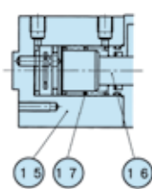
CKA-20AS 常闭型
