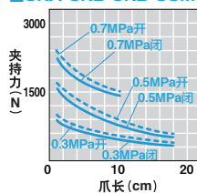
■CKA·CKB·CKD-60MS
